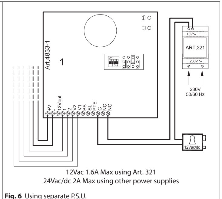
Fig. 6 Using separate P.S.U.
