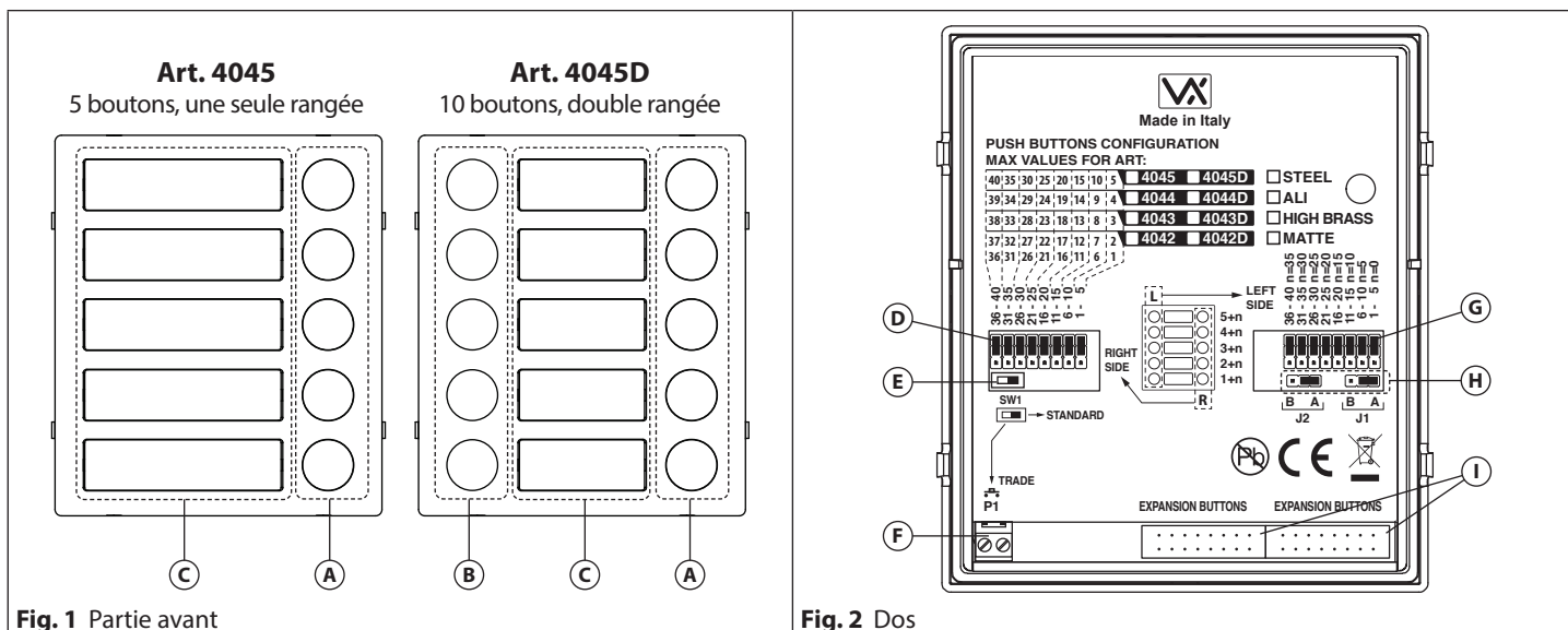
Fig. 1 Partie avant
