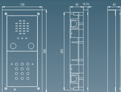
2 push button panel Posto esterno a 2 pulsanti Poste extérieur a 2 boutons Placa exterior 2 botones
